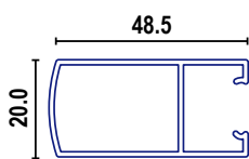
1766 TRASLAPE
