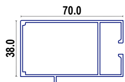
ALN 705 ENGANCHE
