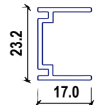
ALN 403 ADAPTADOR
