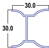
ALN 827 ADAPTADOR
