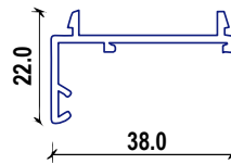
ALN 175 ADAPTADOR
