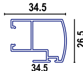
1767 ENGANCHE
