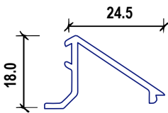
ALN 177 PISAVIDRIO
