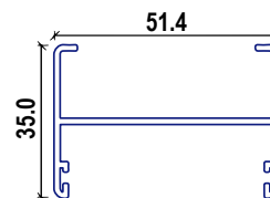
ALN 840 ADAPTADOR
